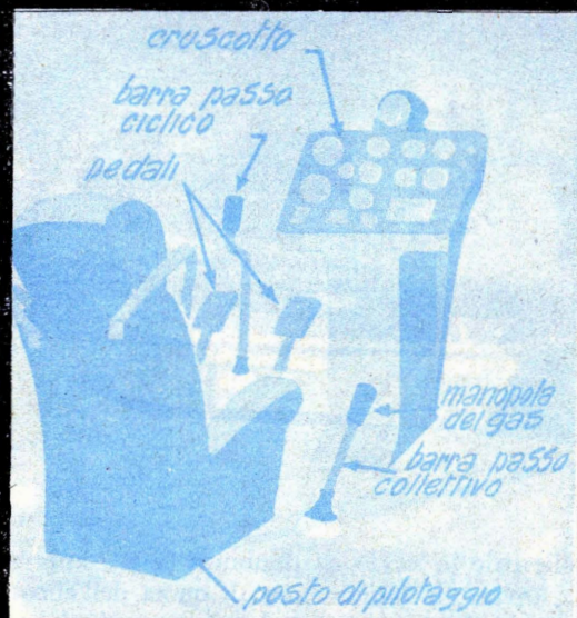
Fig. 1 - Schema della parte anteriore di un elicottero.
