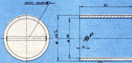
TAMPONE PER MONTAGGIO CAMERA PARACADUTI N°1 PEZZO MATERIALE A00
