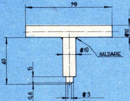
TONDINO PRESSAGGIO MOLLA
