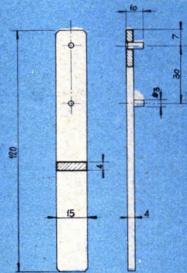
CHIAVE PER MONTAGGIO CAMERA PARACADUTI N°1 PEZZO MATERIALE A37
