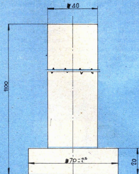
TAMPONE PER COMPRIMERE LA MICROGRANA
