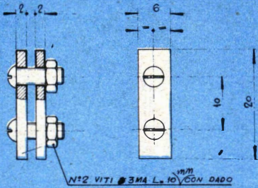
REGOLATORE PASSAGGIO OSSIGENO MAT. A00
