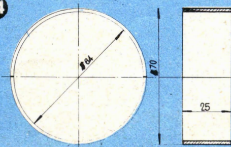
ANELLO IN DUE META MAT. A42
